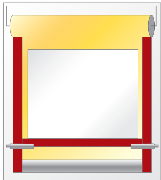
mit Aussteifung, Seitenschienen und Windriegel
